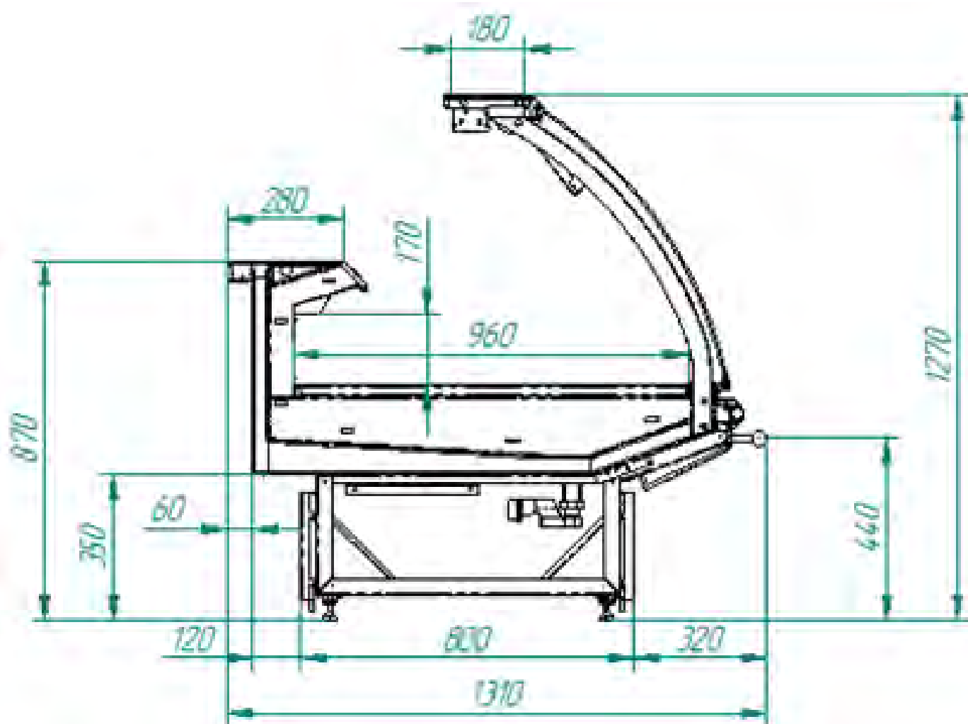
Габаритные размеры
